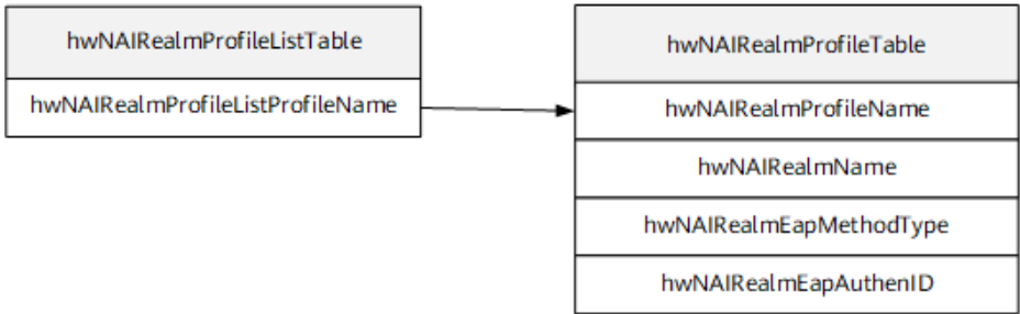
图 141-13 hwNAIRealmProfileListTable 和 hwNAIRealmProfileTable 的表间关系
