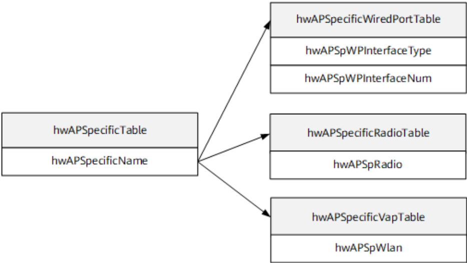
图 141-3 hwAPSpecificTable、hwAPSpecificWiredPortTable、hwAPSpecificRadioTable 和 hwAPSpecificVapTable 的表间关系
