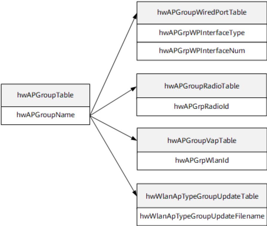
图 141-1 hwAPGroupTable、hwAPGroupWiredPortTable、hwAPGroupRadioTable、hwAPGroupVapTable 和 hwWlanApTypeGroupUpdateTable 的表间关系图
